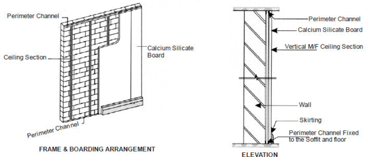
Fig. 9.28 : Wall Panelling
